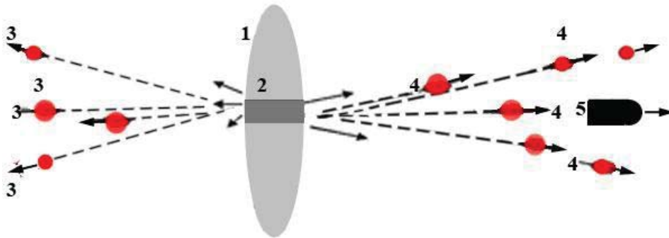
Рис. 1. Выбивание конуса брызг крови пульей: 1 – биообъект; 2 – раневой канал; 3 – брызги крови, образующие «обратный» конус; 4 – брызги крови, образующие «прямой» конус; 5 – пуля
