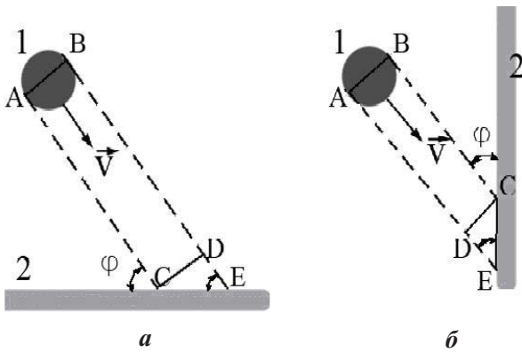
Рис. 2. Падение брызг крови на поверхность: а – горизонтальную; б – вертикальную
