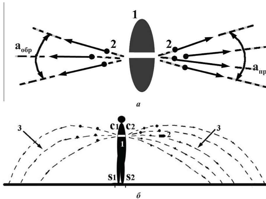
Рис. 3. Формирование прямого и обратного конусов брызг крови при пробитии пулей биомишени: a – вид сверху (1 – биомишень, 2 – выбитые брызги крови, a_{обр} и a_{пр} – углы разлета брызг крови в горизонтальной плоскости); б – вид сбоку ( C_1 , C_2 – точки вылета брызг крови обратного и прямого конуса соответственно (входное и выходное отверстие раневого канала соответственно), S_1 и S_2 – проекции точек вылета C_1 и C_2 на горизонтальную плоскость, 1 – биомишень, 2 – снаряд, 3 – траектории полета выбитых частичек крови)
