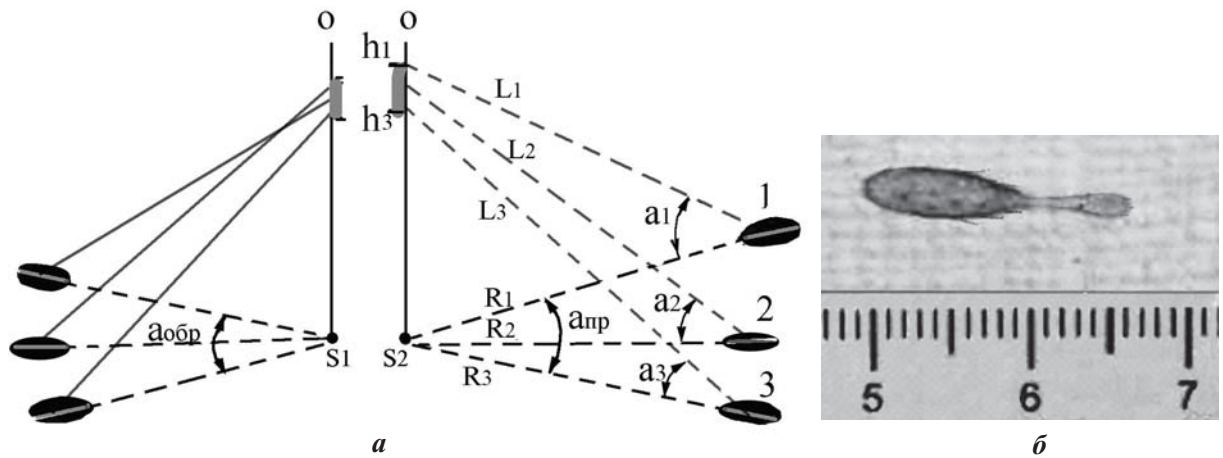
Рис. 4. Пятна брызг крови, выбитых снарядом, на горизонтальной поверхности: a – 1, 2, 3 – пятна брызг крови; a_{обр} и a_{пр} – углы разлета брызг крови в горизонтальной плоскости; R_1 , R_2 , R_3 – направления вылета каплей крови; L_1 , L_2 , L_3 – линии подлета каплей крови к преграде; a_1 , a_2 , a_3 – углы встречи каплей крови с преградой; h_1 – h_3 – интервал высот, на котором располагался раневой канал в момент ранения; б – пятно частицы крови, выбитой пулей из имитатора биологических тканей, на смачиваемой поверхности
