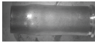
Рис. 4. Бутылочная форма гильзы спортивного пистолетного патрона калибра 7,62 мм, штатного к ТОЗ 49, после выстрела из пистолета «Маузер К 96» образца 1896 г.
